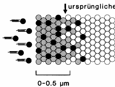
Ionenstrahlmischen
