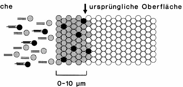
Ionenstrahlgestützte Beschichtung
